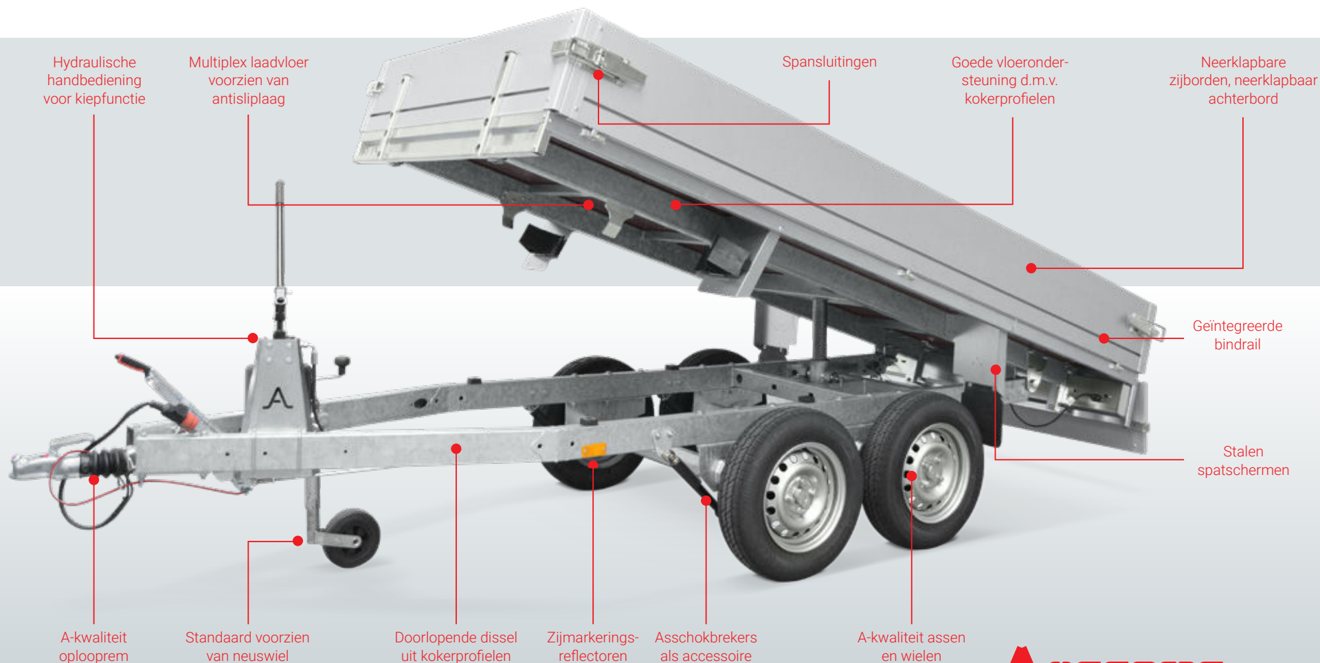
Disselprofielen lopen door tot achterzijde laadbak
